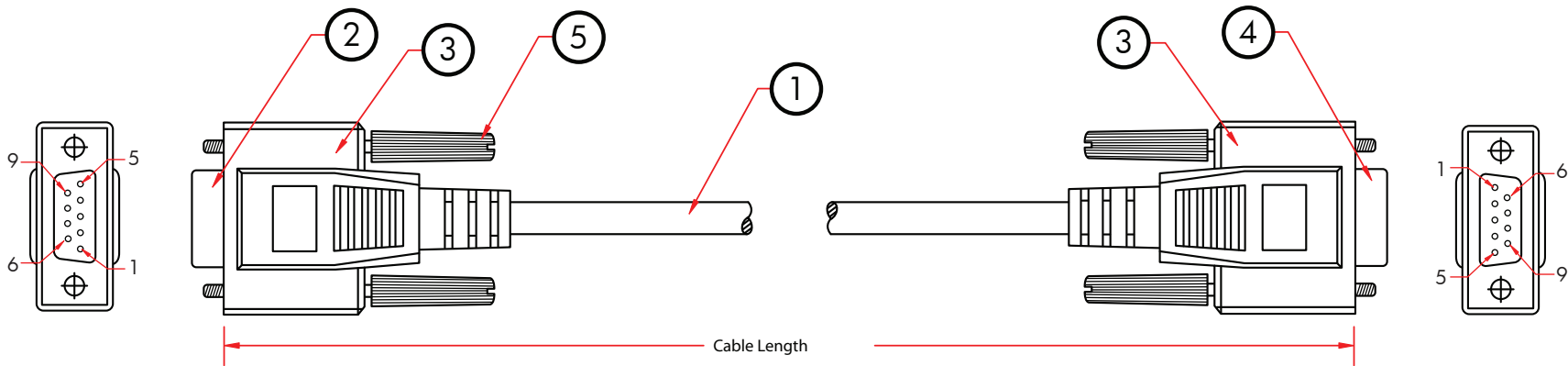
DB9 / F
